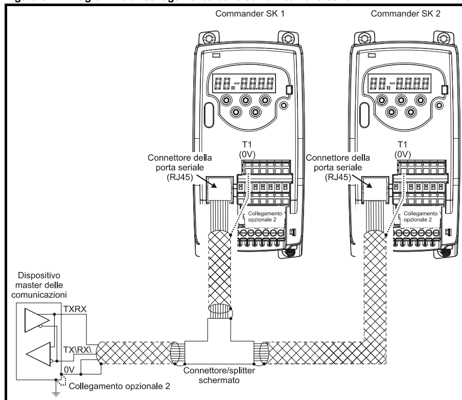
Figura 5-1 Diagramma di collegamento delle comunicazioni seriali
