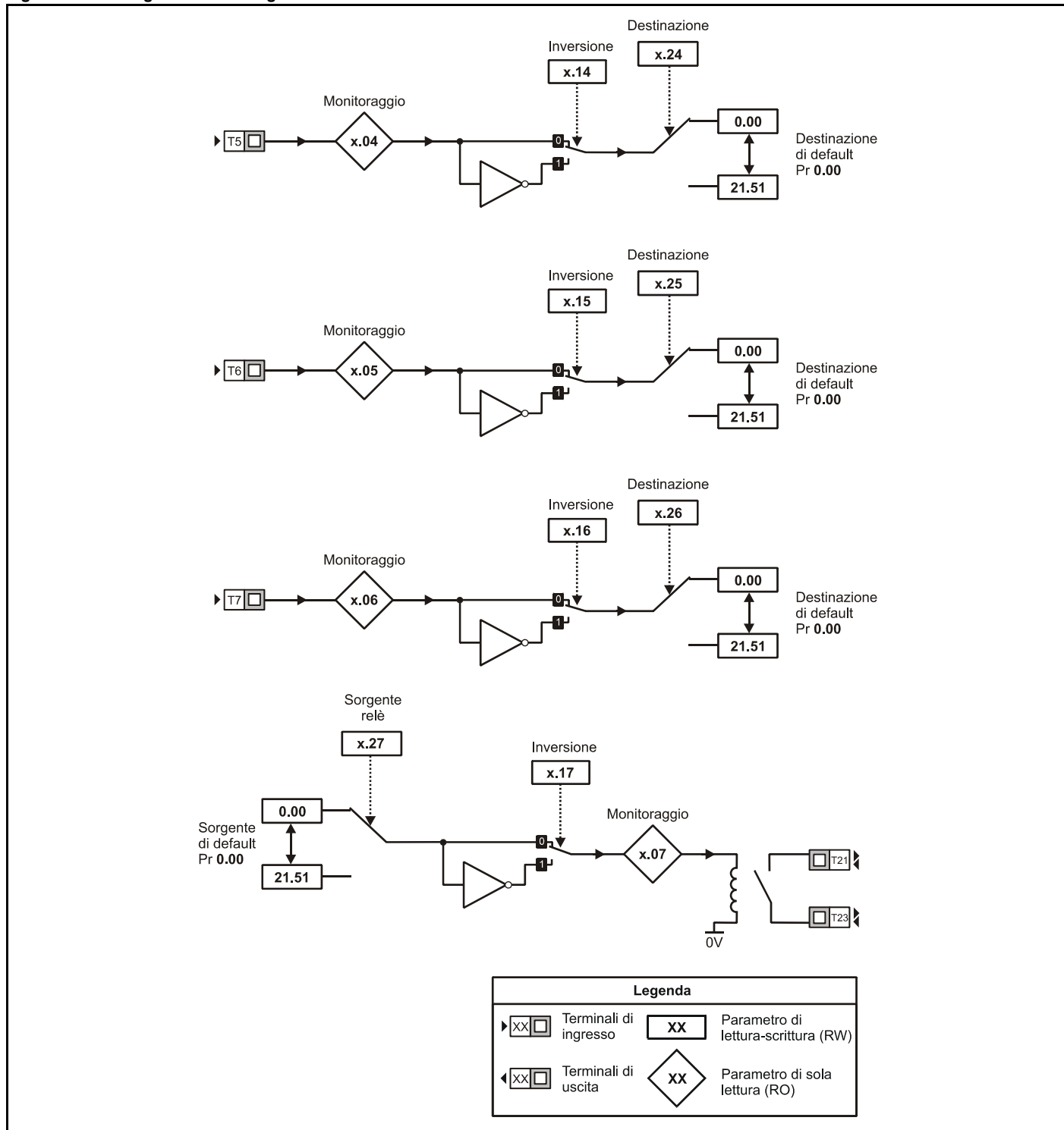
Figura 10-44 Diagramma della logica del Menu 15A*
