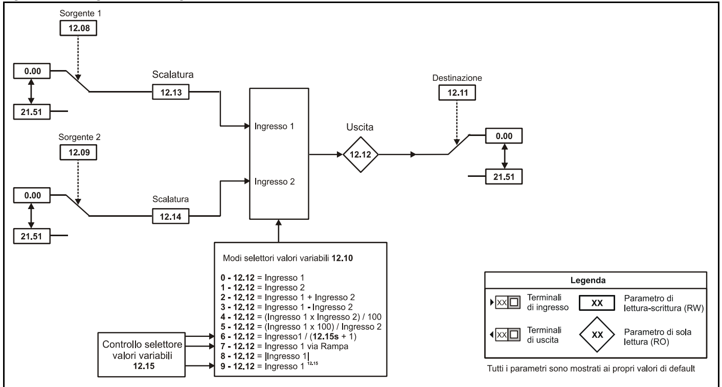
Figura 10-38 Diagramma della logica del Menu 12C
